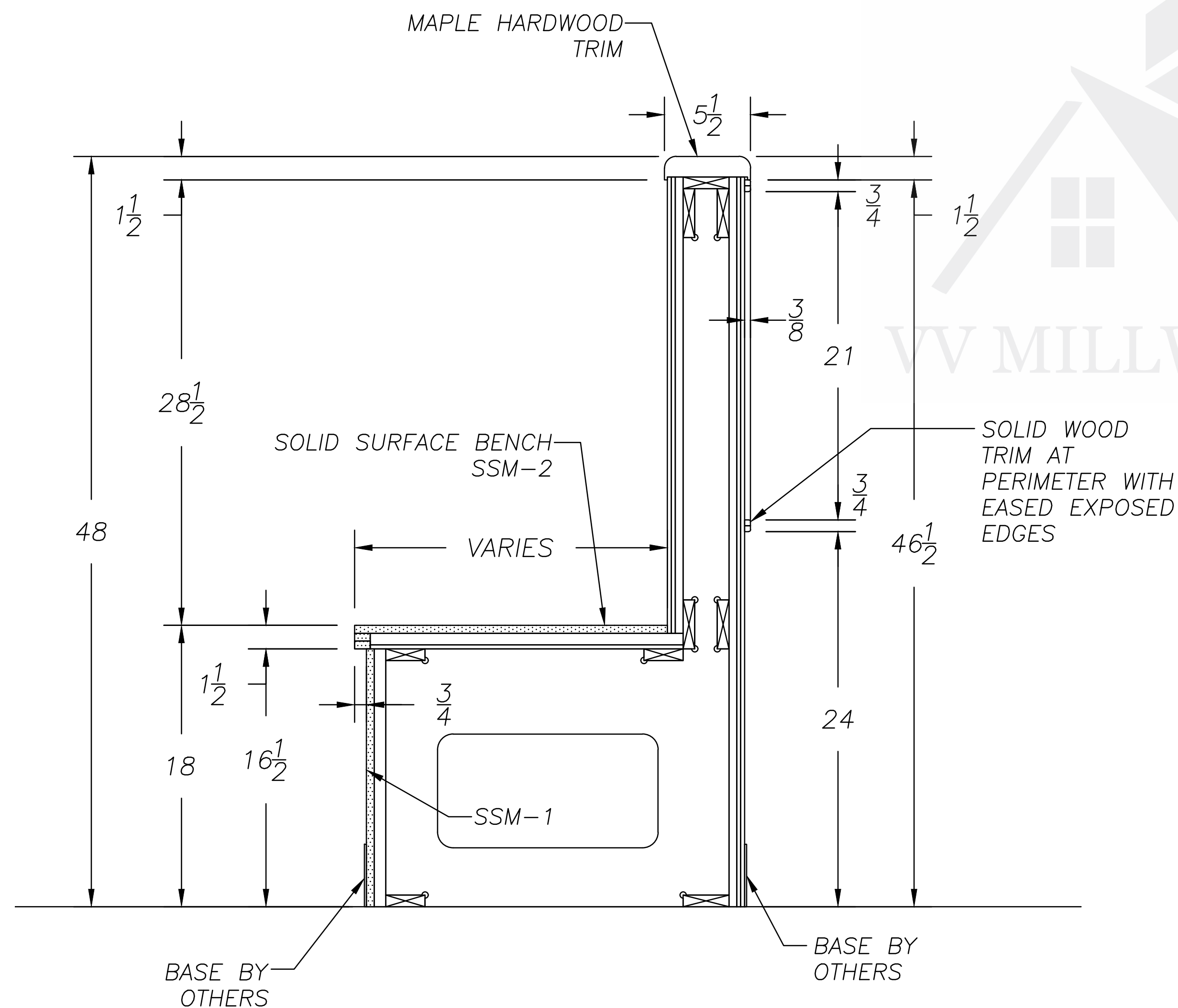
SECTION 1 SCALE: 1"=1'0"
