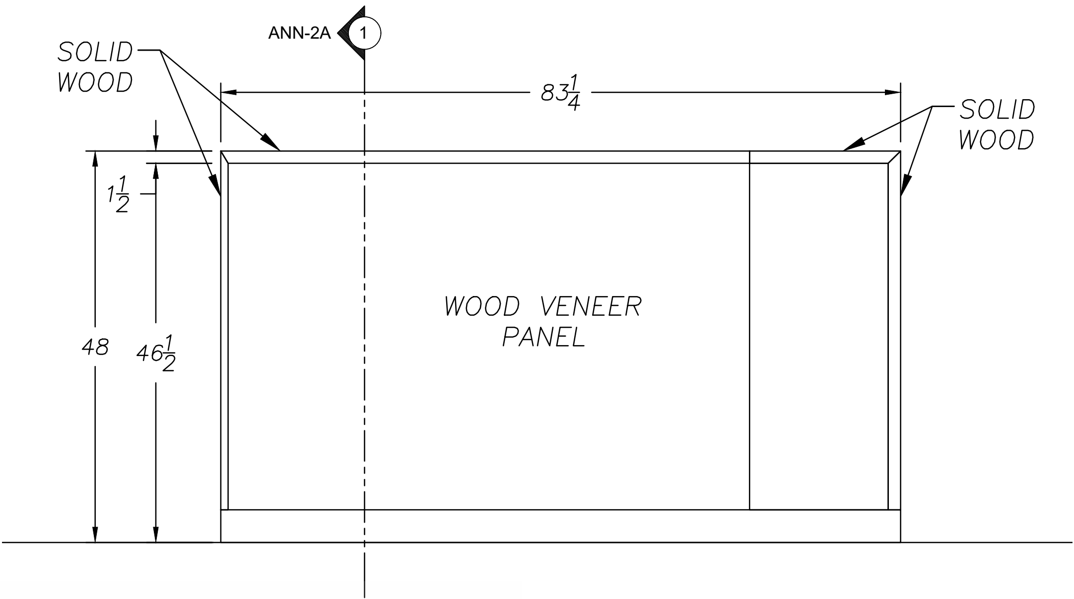
ELEVATION 4 SCALE: 1/2"=1'0"
