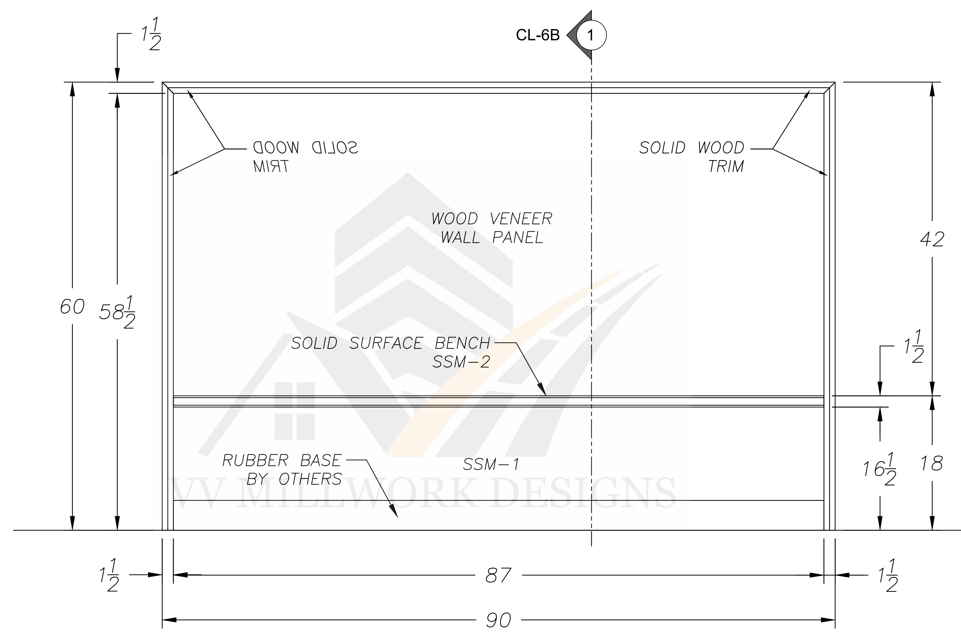
ELEVATION 1 SCALE: 3/4"=1'0"
