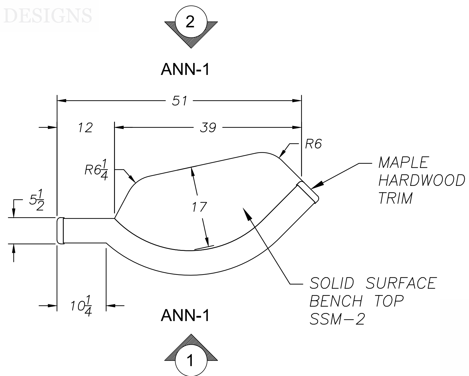
PLAN SCALE: 1/2"=1'0"
