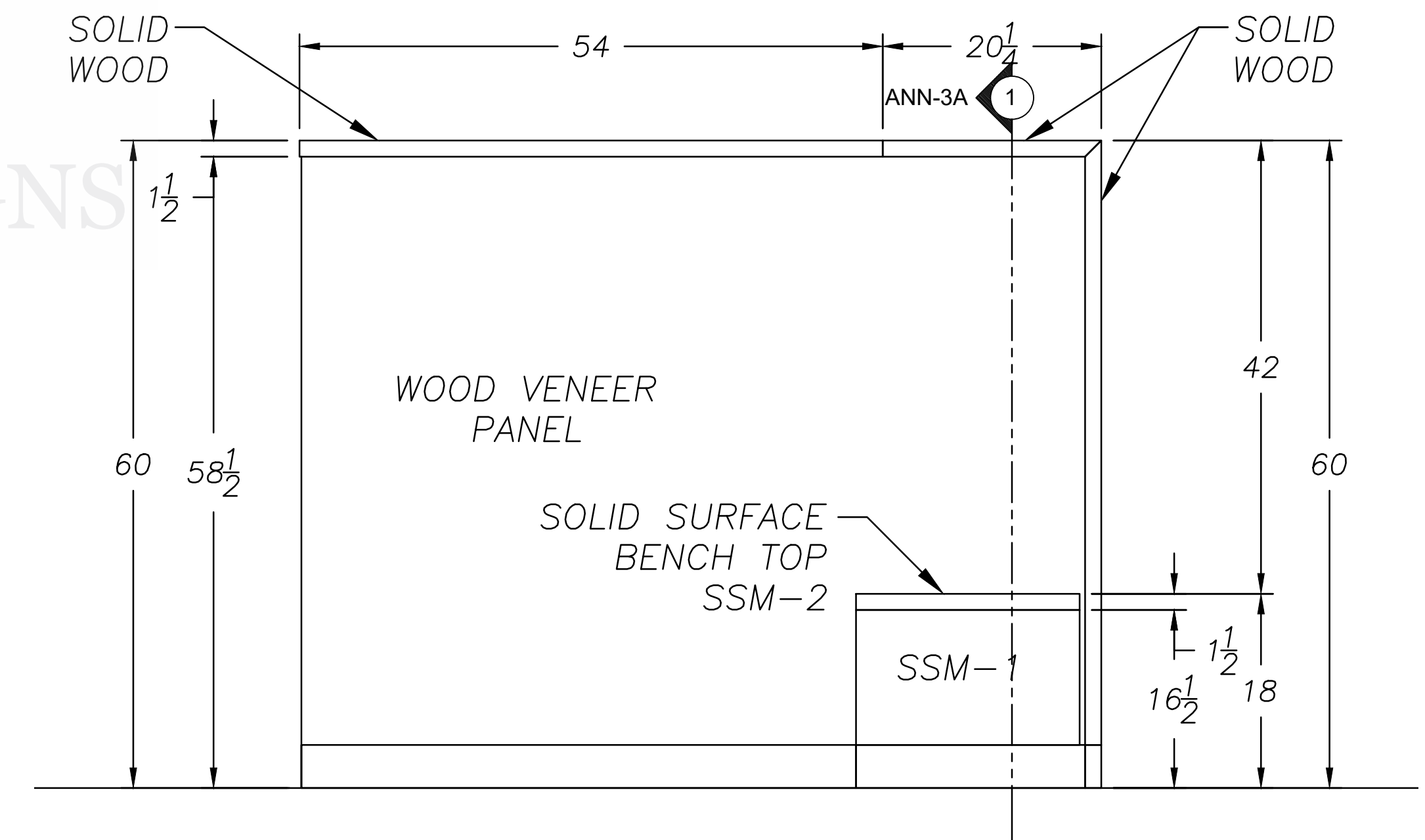
ELEVATION 3 SCALE: 1/2"=1'0"
