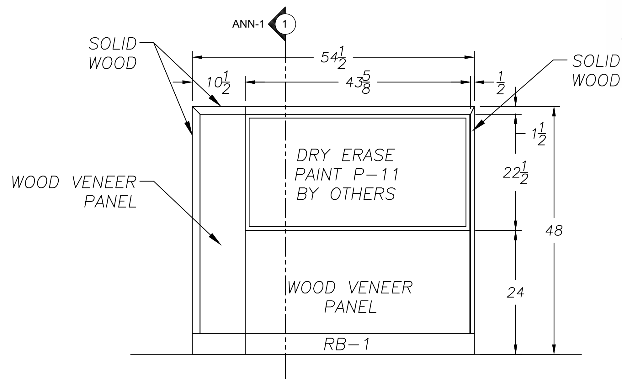
ELEVATION 1 SCALE: 1/2"=1'0"
