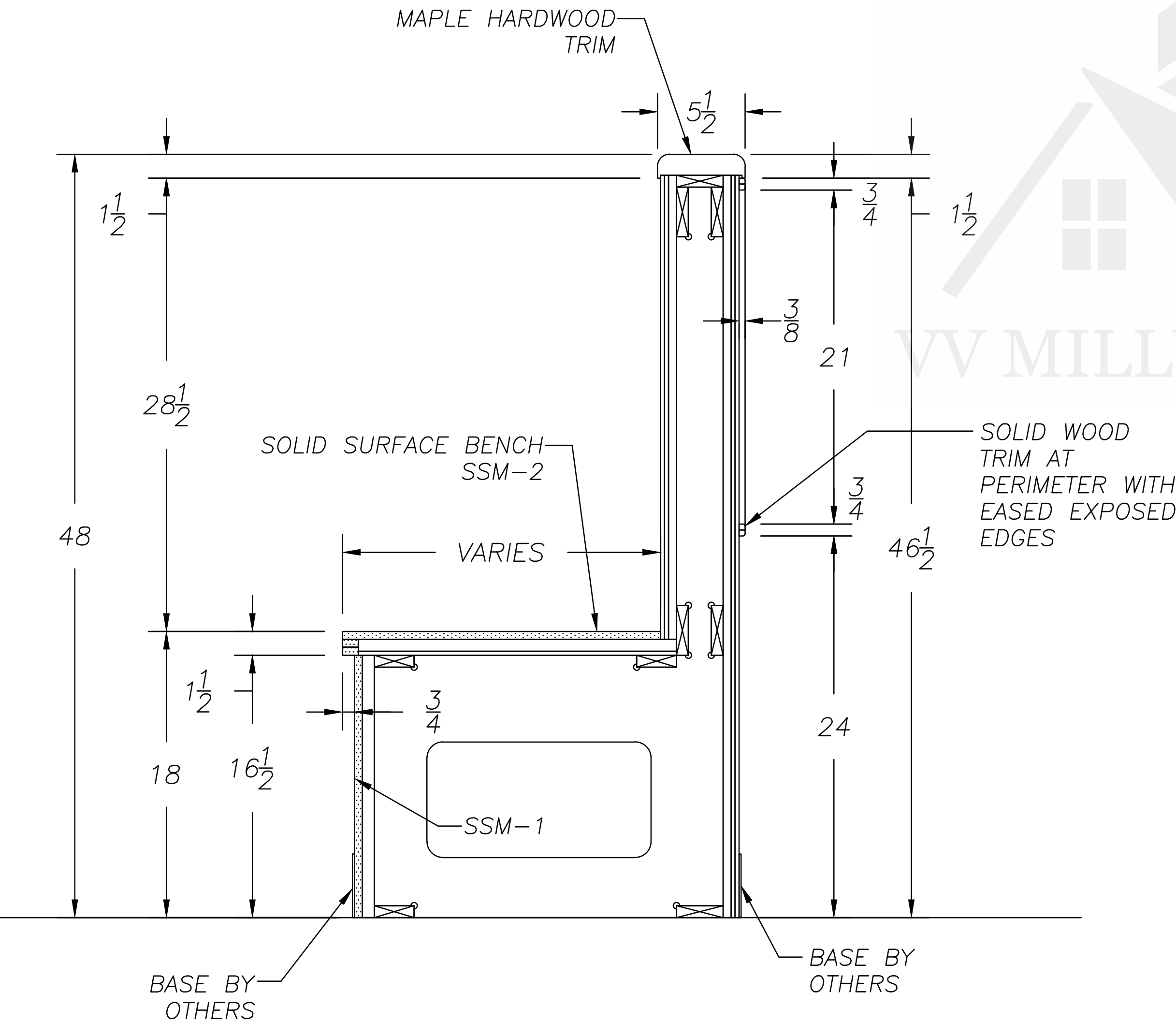
SECTION 1 SCALE: 1"=1'0"
