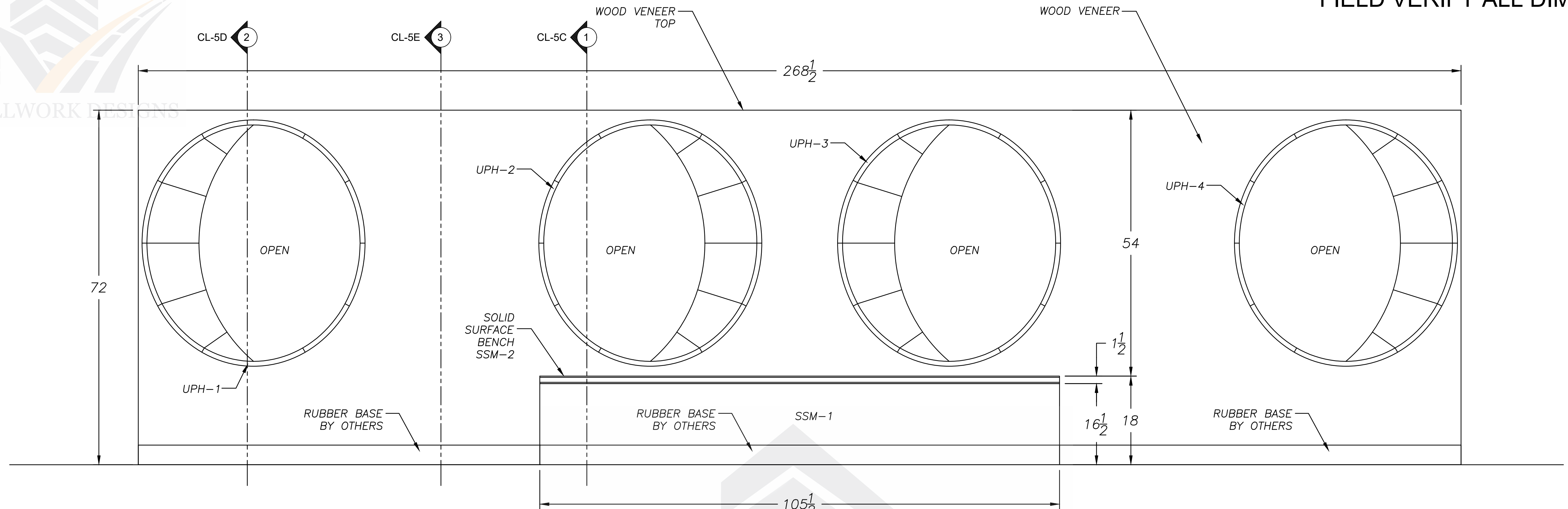
ELEVATION 1 SCALE: 1/2"=1'0"
