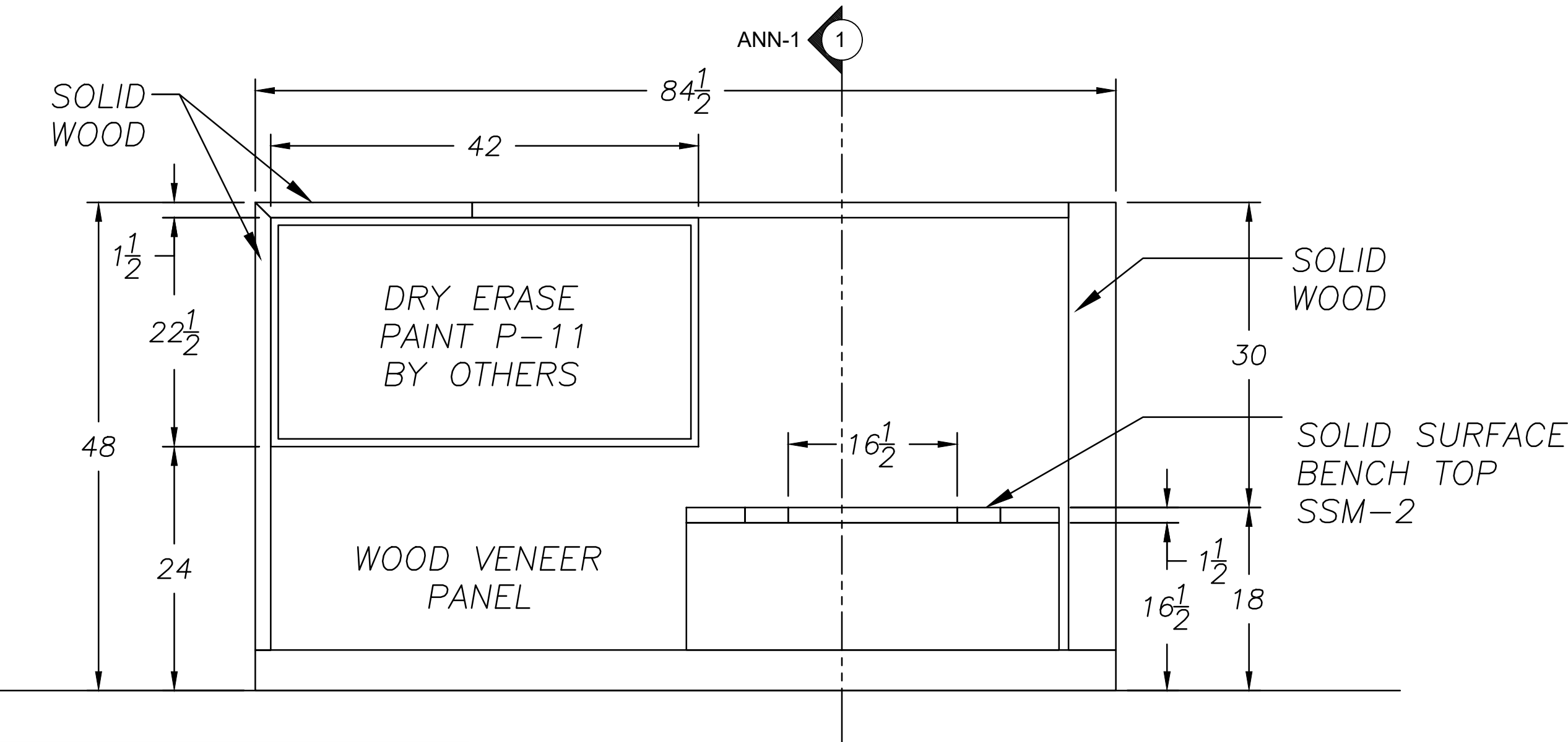
ELEVATION 4 SCALE: 1/2"=1'0"
