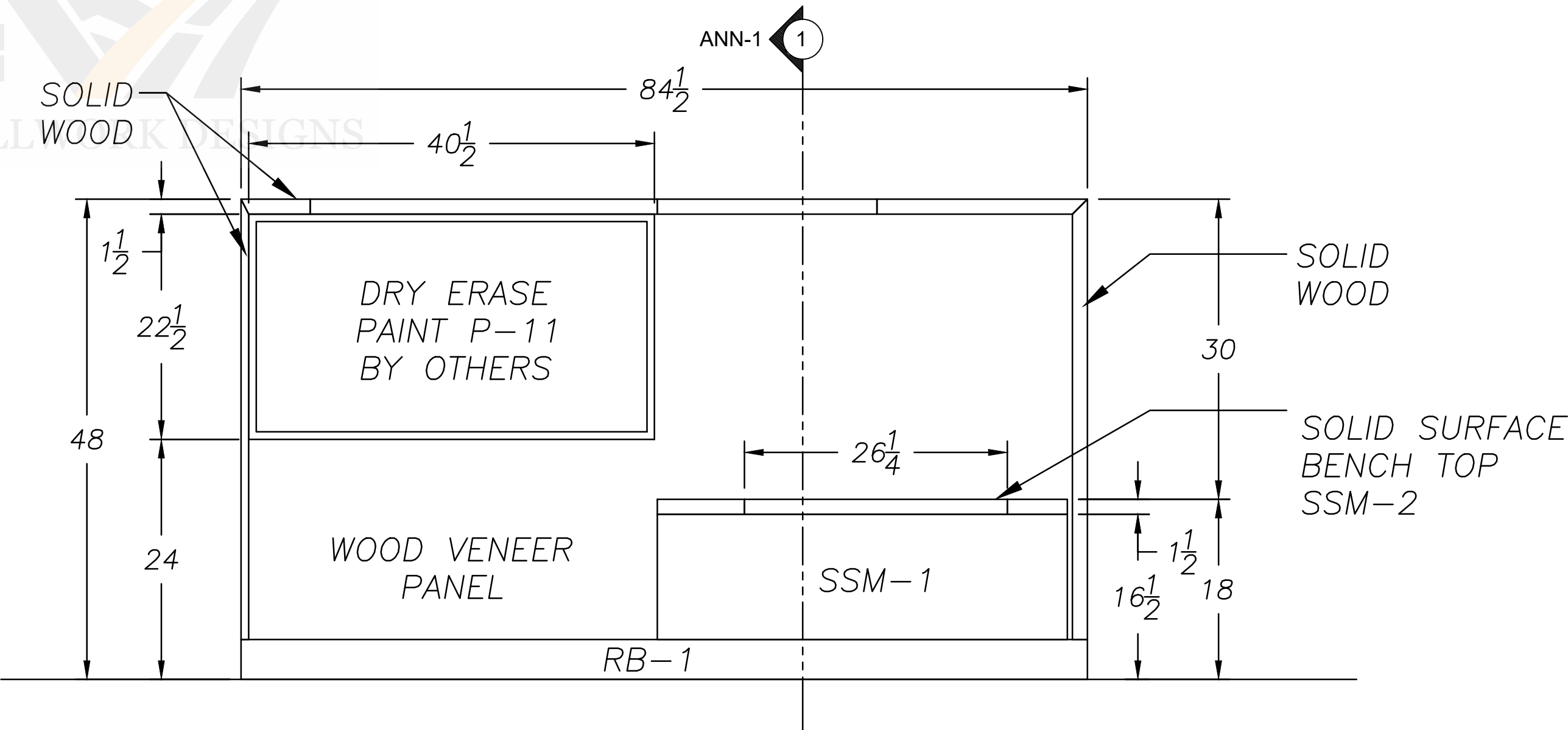
ELEVATION 3 SCALE: 1/2"=1'0"
