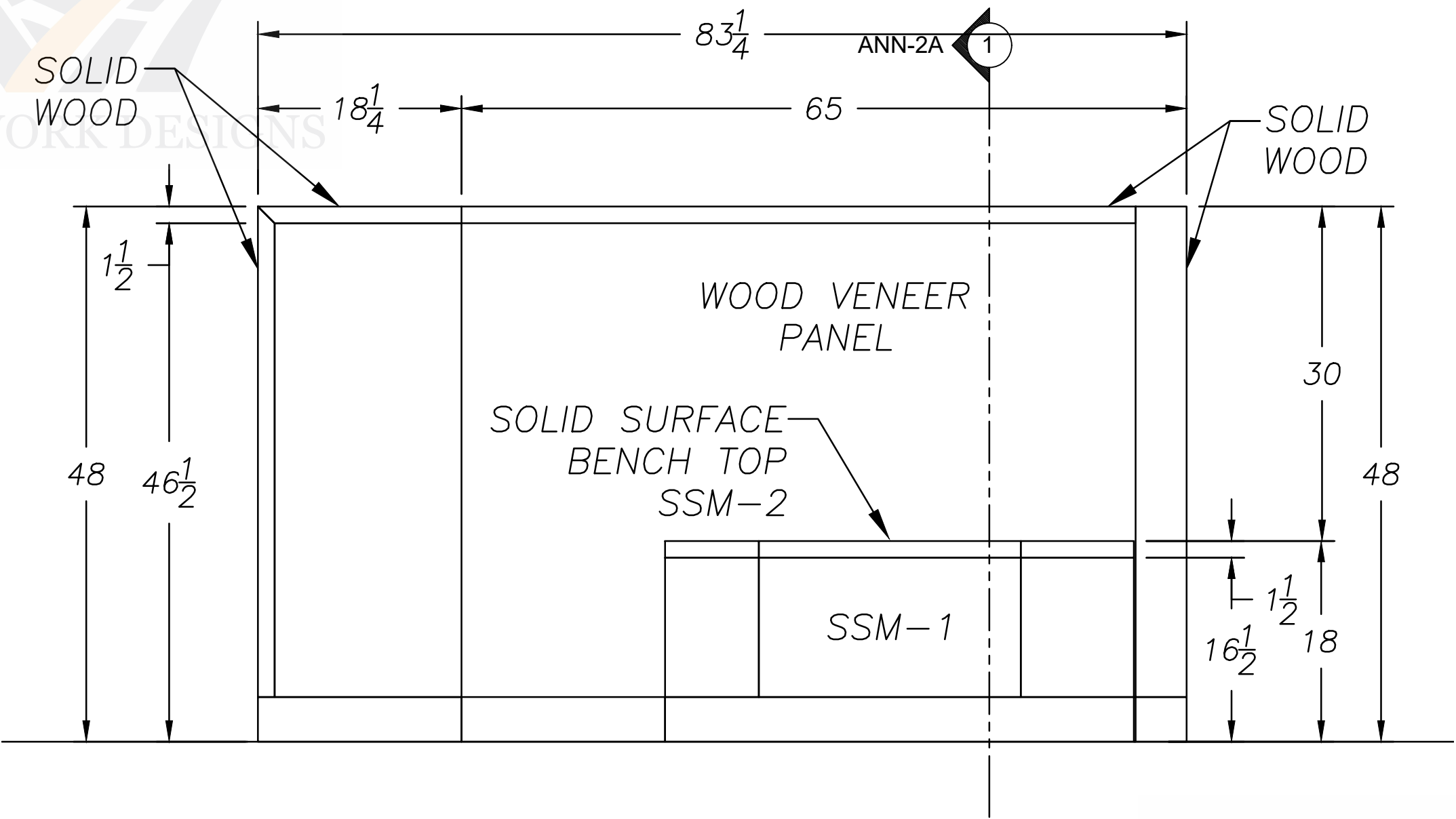
ELEVATION 3 SCALE: 1/2"=1'0"
