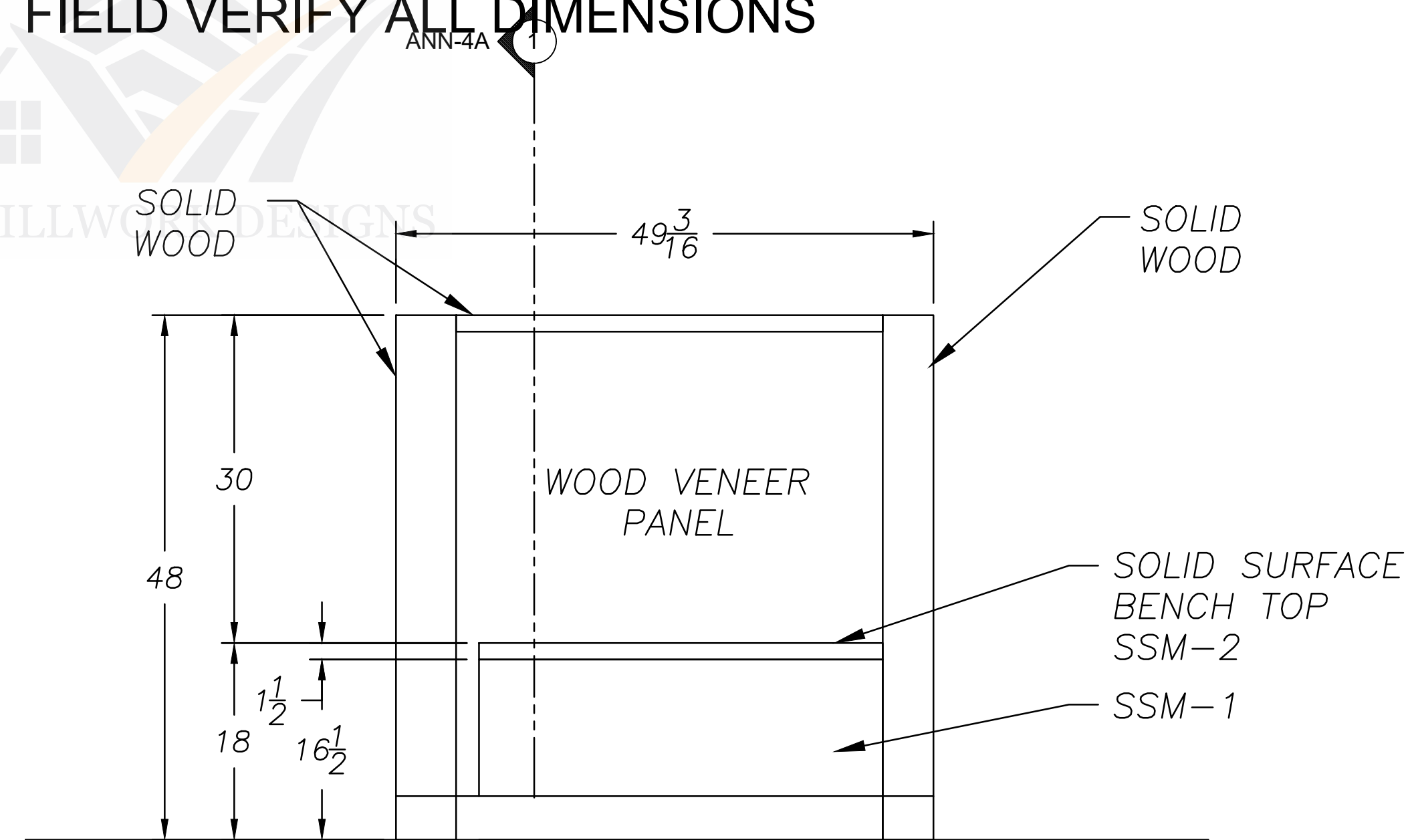
ELEVATION 4 SCALE: 1/2"=1'0"
