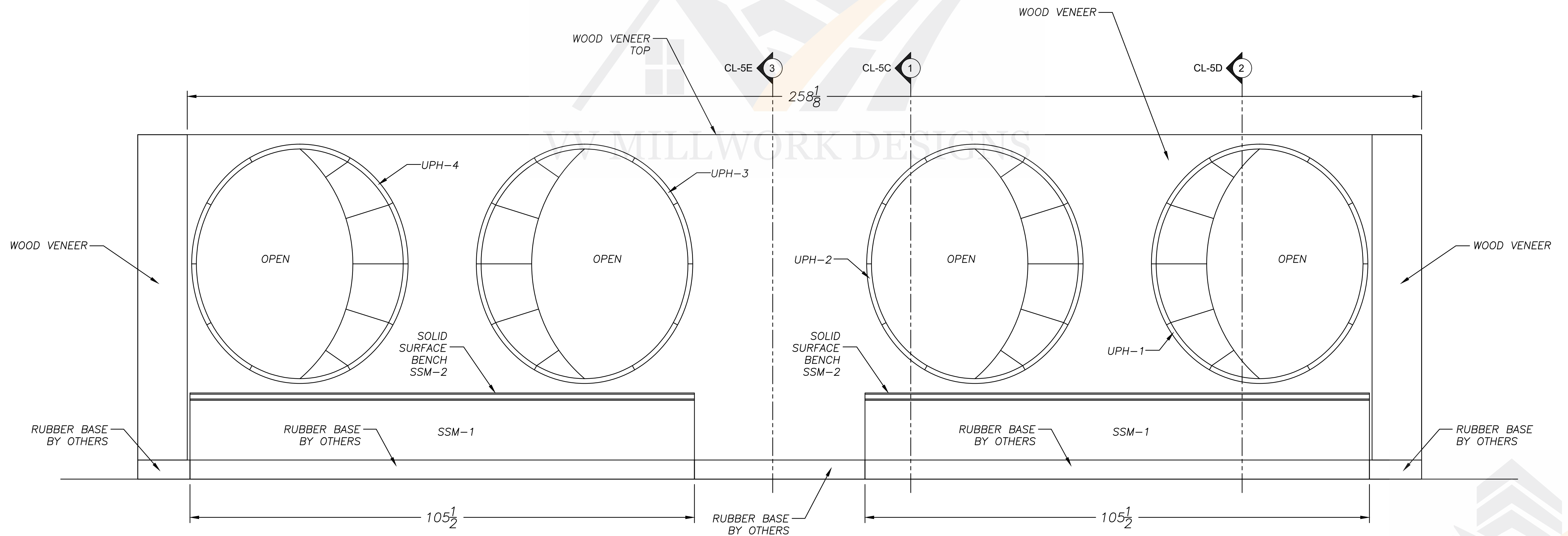
ELEVATION 2 SCALE: 1/2"=1'0"
