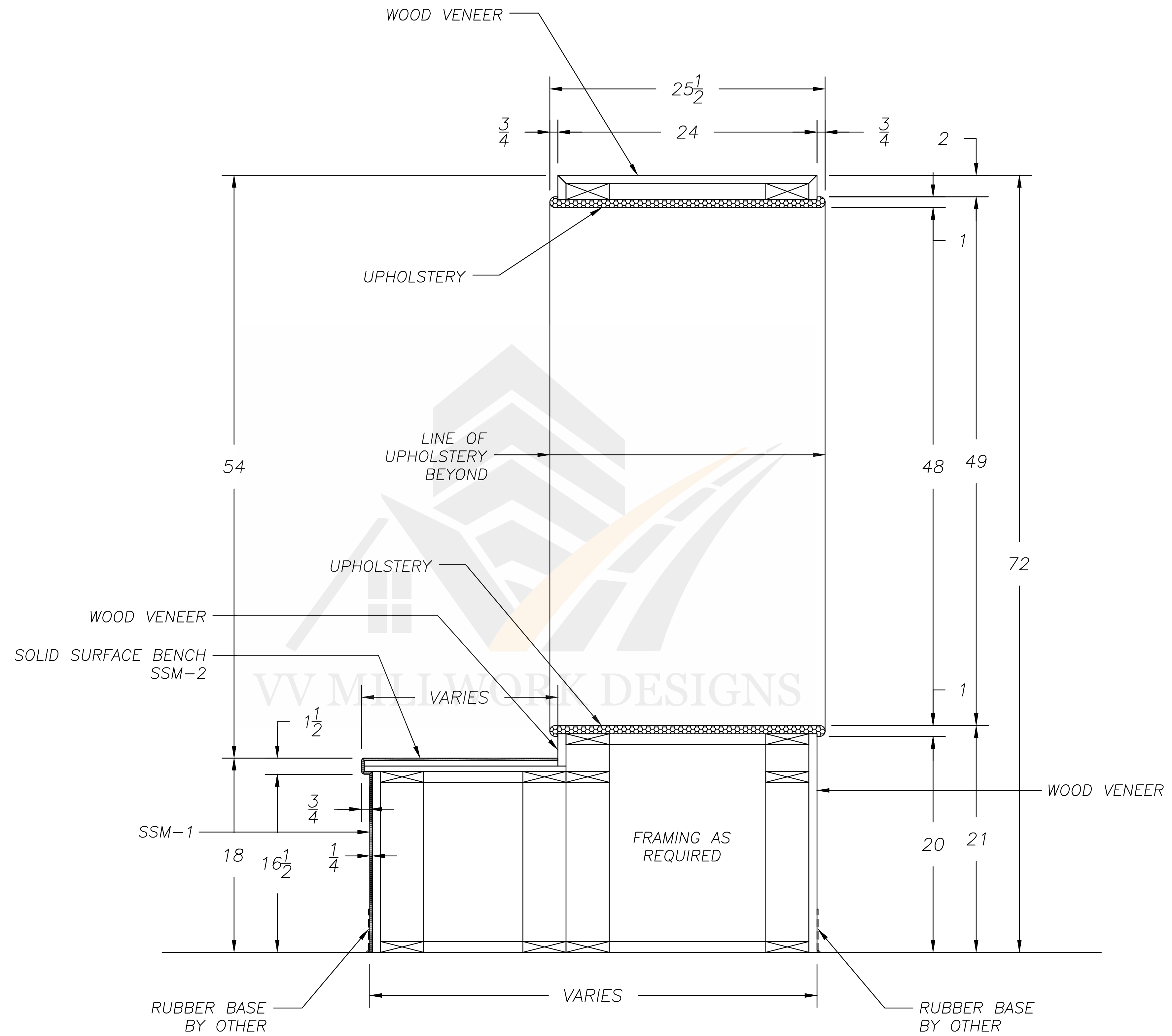
SECTION 2 SCALE: 1"=1'0"
