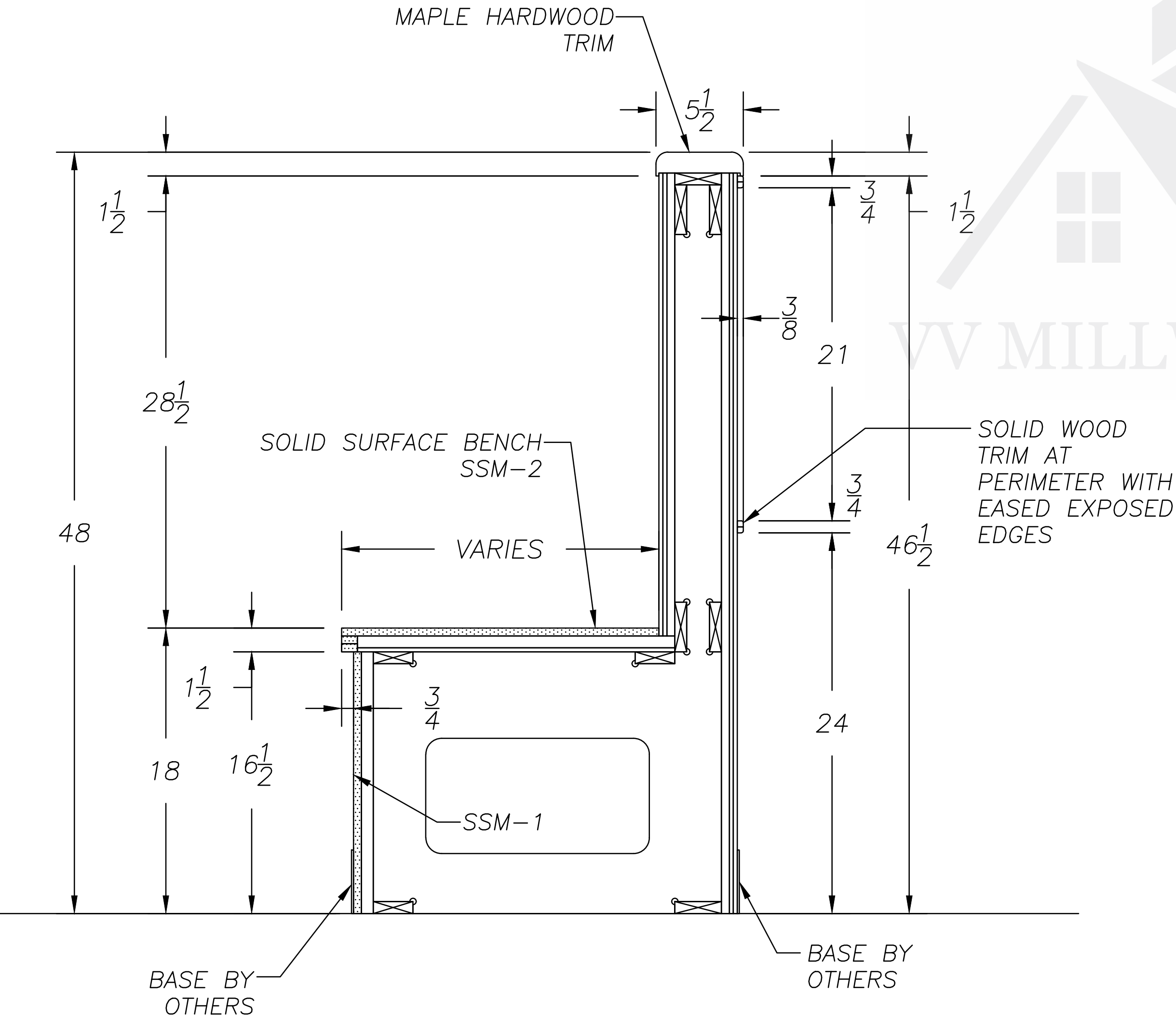
SECTION 1 SCALE: 1"=1'0"
