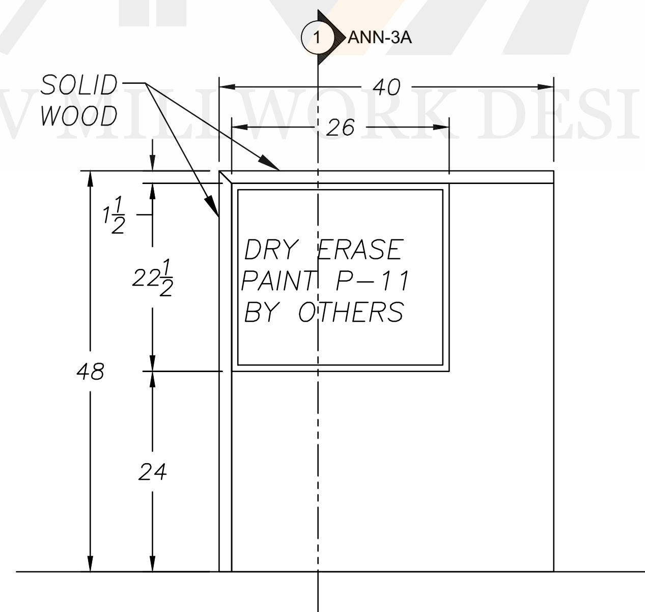
ELEVATION 2 SCALE: 1/2"=1'0"
