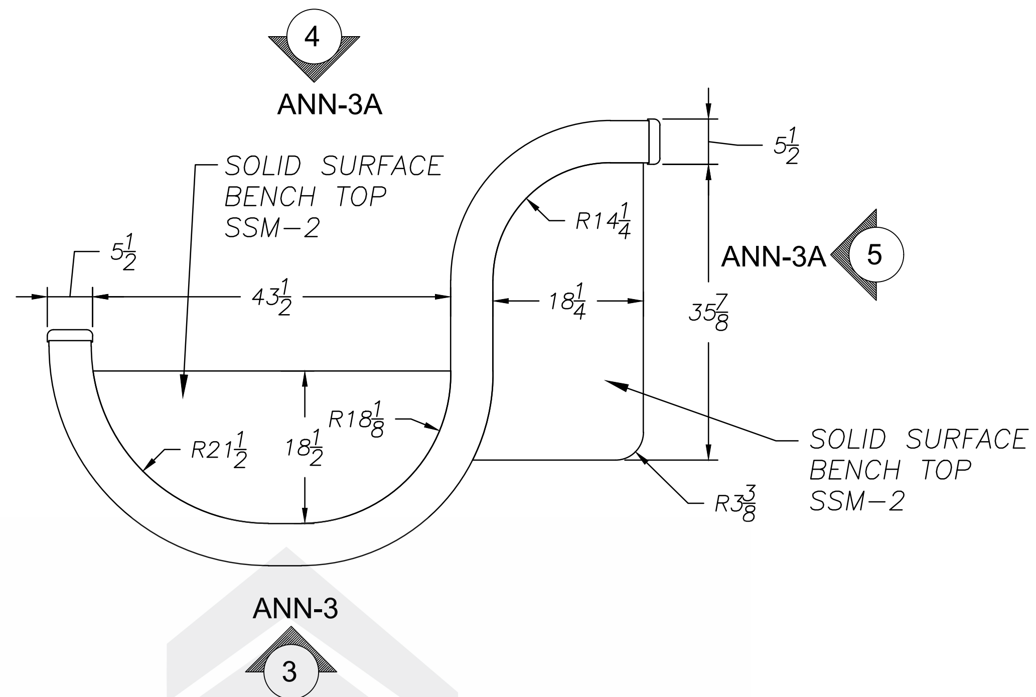
PLAN SCALE: 1/2"=1'0"
