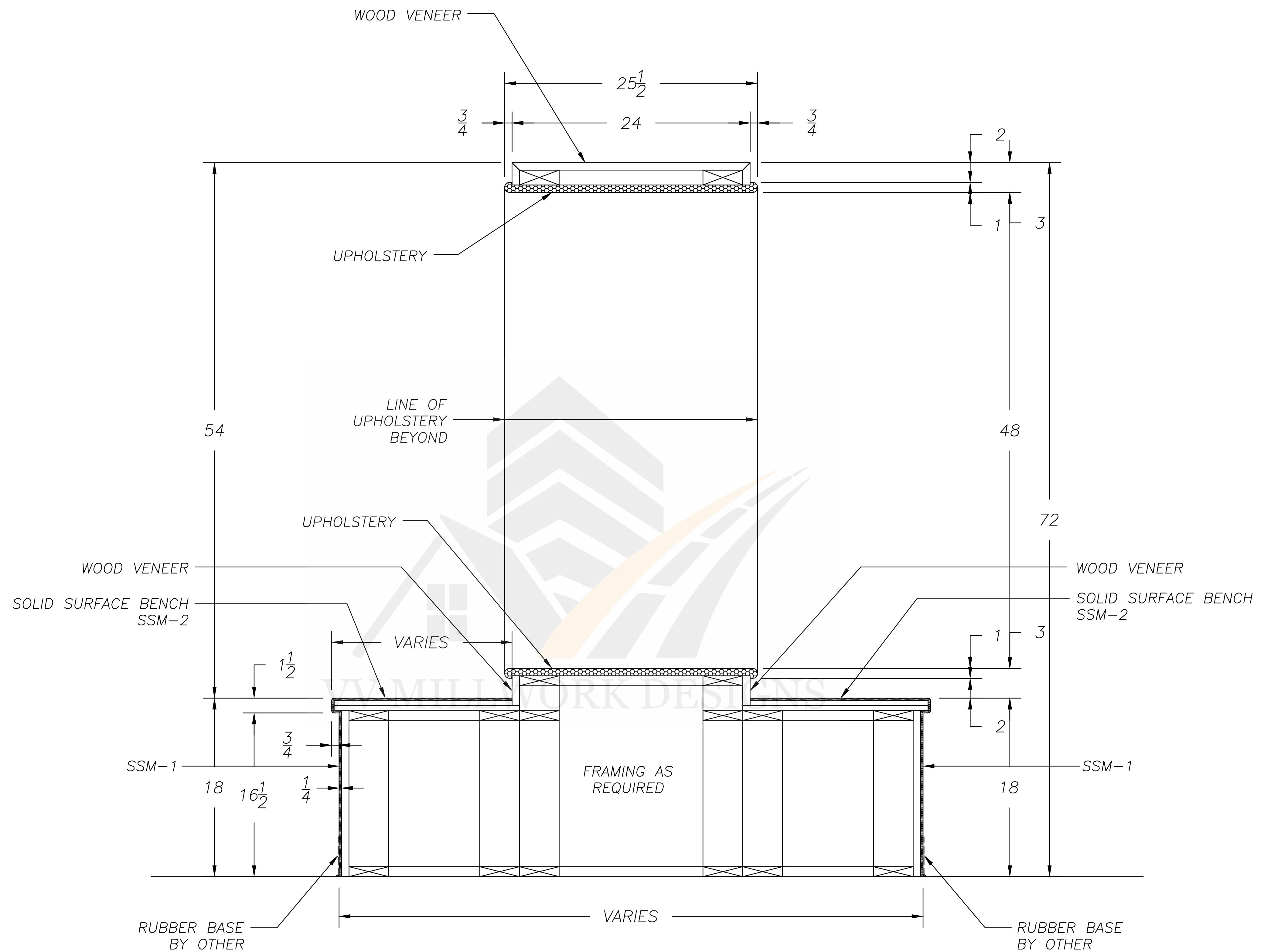
SECTION 1 SCALE: 1"=1'0"
