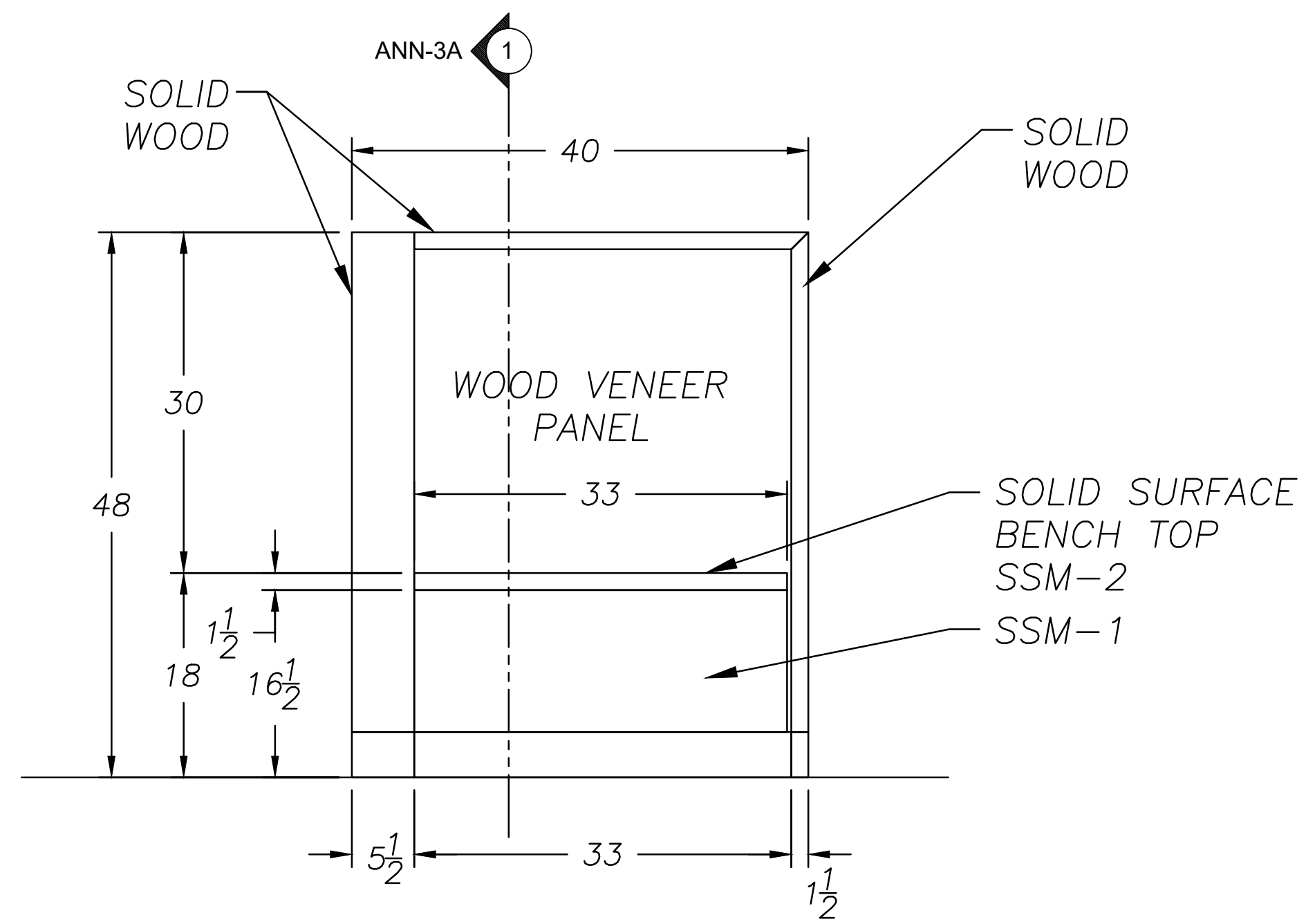
ELEVATION 1 SCALE: 1/2"=1'0"
