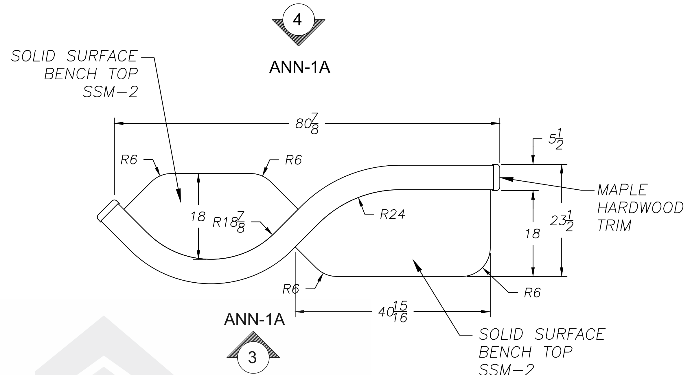
PLAN SCALE: 1/2"=1'0"
