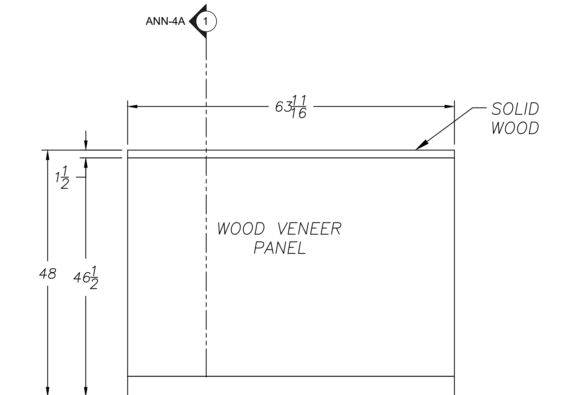
ELEVATION 5 SCALE: 1/2"=1'0"
