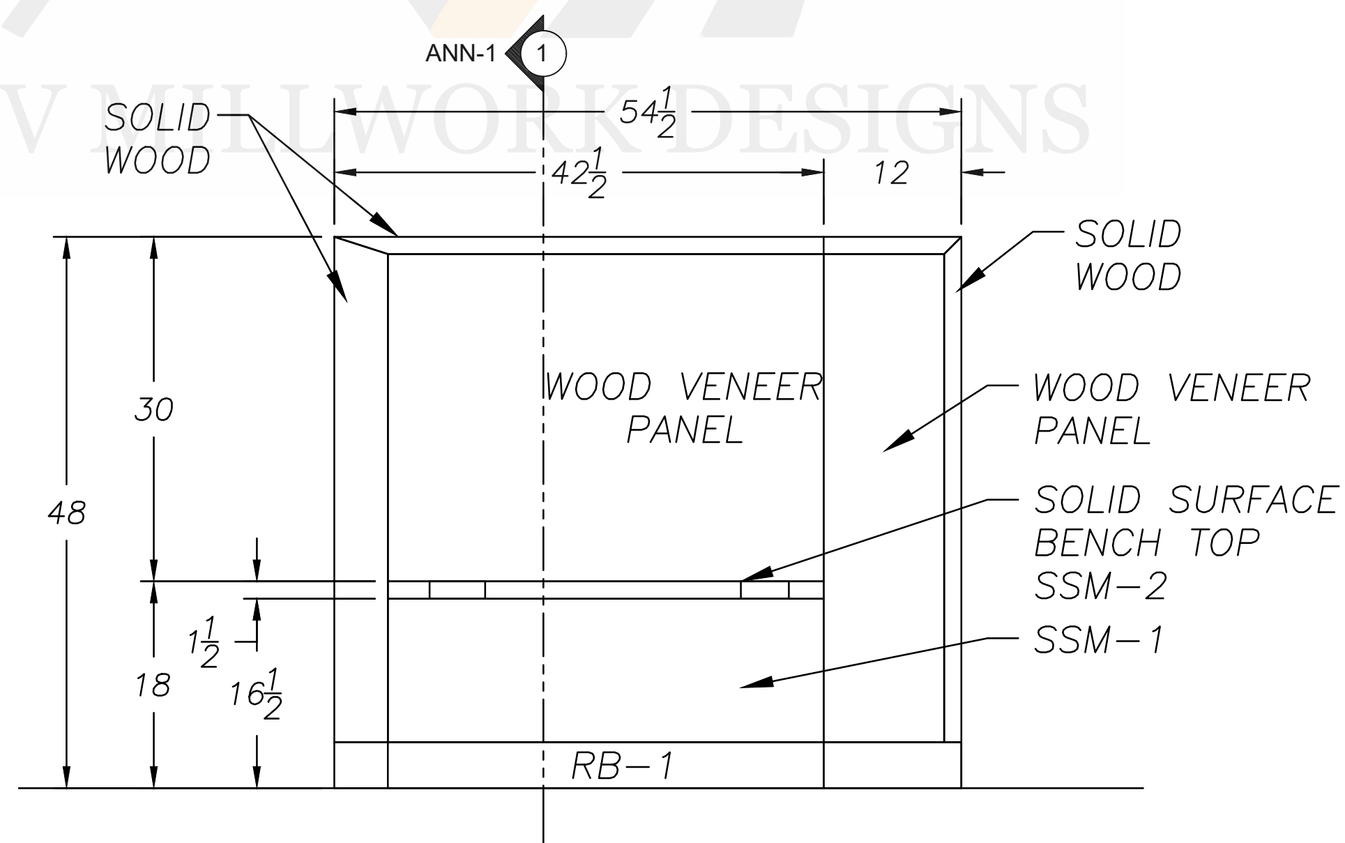
ELEVATION 2 SCALE: 1/2"=1'0"
